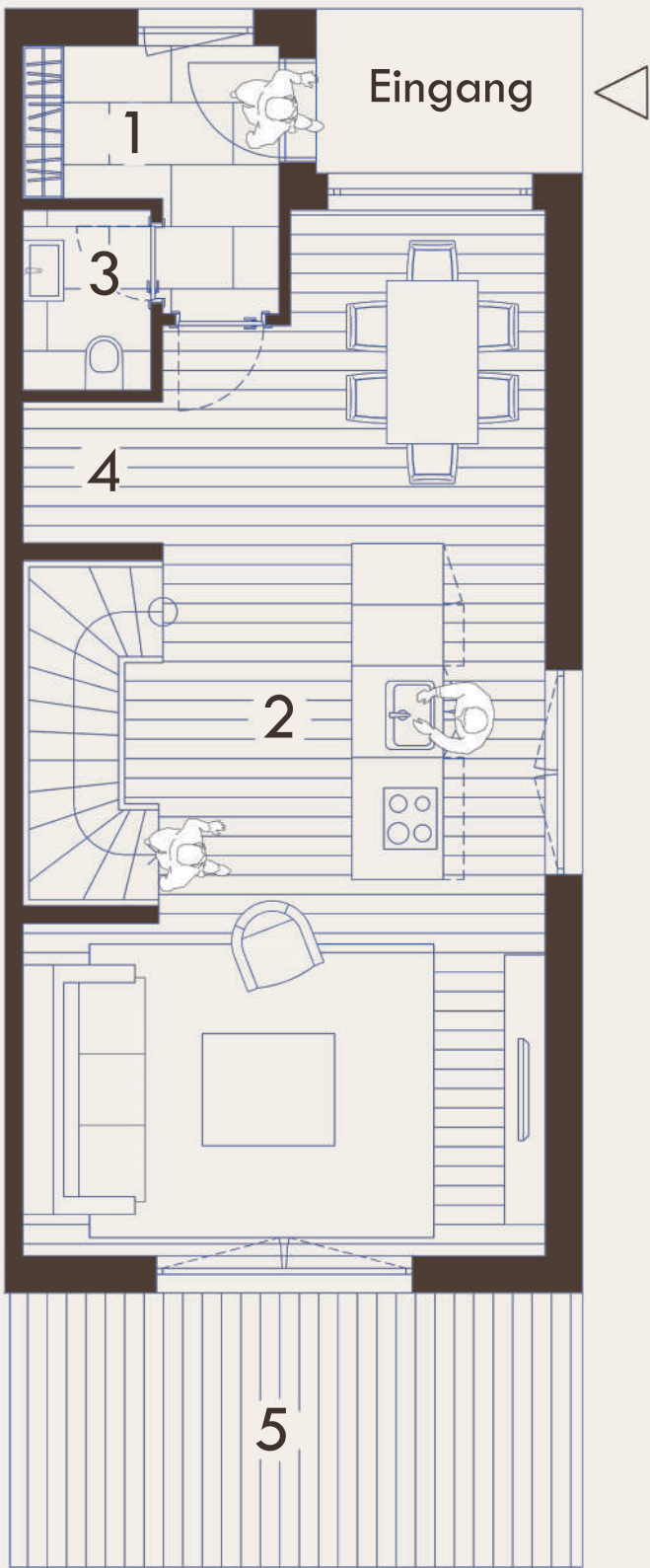
Erdgeschossplan
