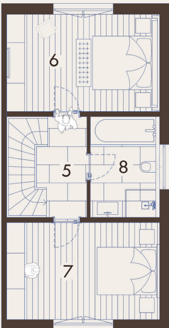
Obergeschossplan
